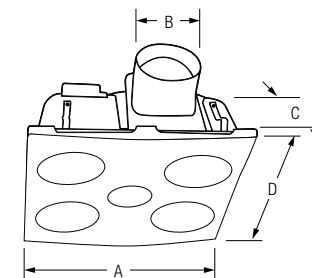
FAN6882 FAN6883
