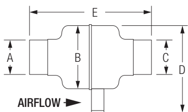
EL100
